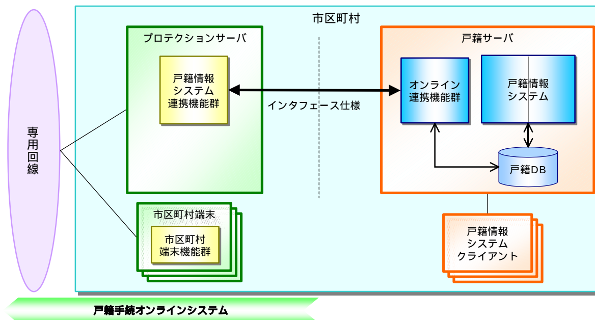
図 6-1 戸籍情報システム共用方式
